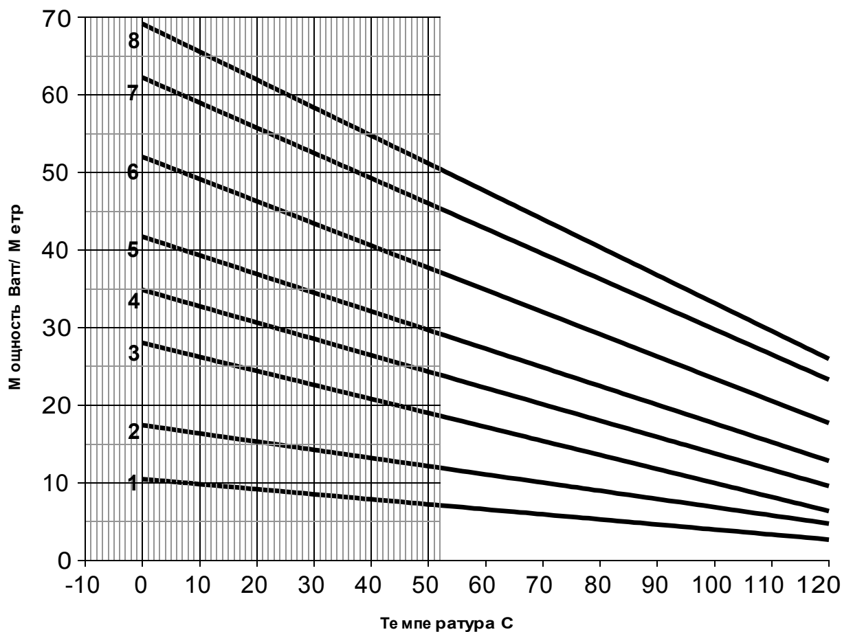
Мощность серии HLT @ 240v
